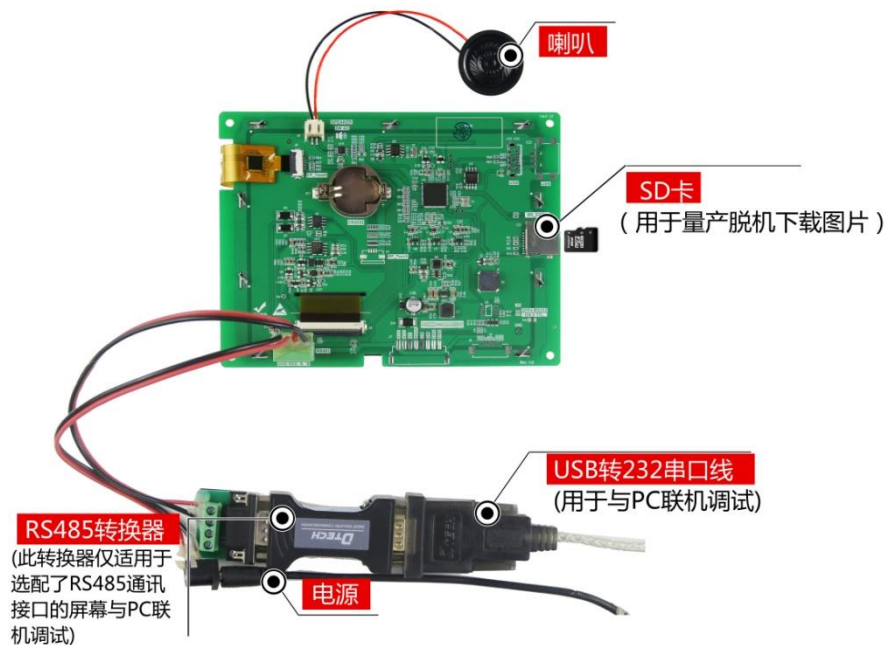
图 1-5 调试工具图
