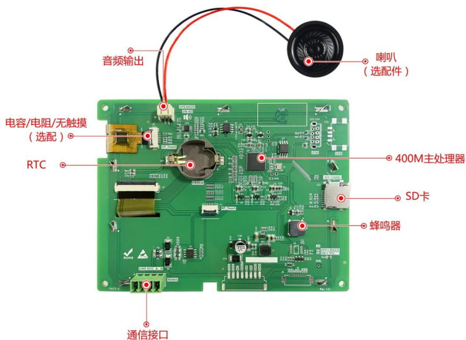
图 1-4 硬件配置图
